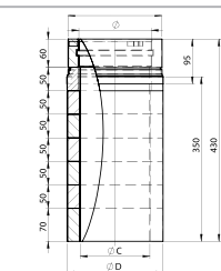
Paspipij / ADWECO1160
