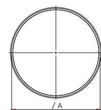
Dichtring - 200 pa / ALBI26
