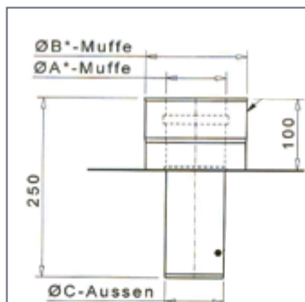
Verloop FLEX/TWIN / ATWIN466
