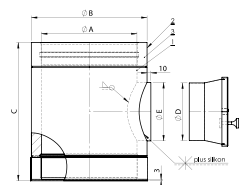
Element met trekregelaar / ADW806
