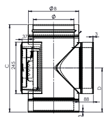
T-Stuk 90° met reinigingsopening / ADWECO309
