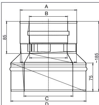
Verloop 100/150 - 130/200 / ATWIN464
