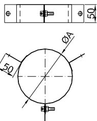
Tuidraad beugel / ADWECO42
